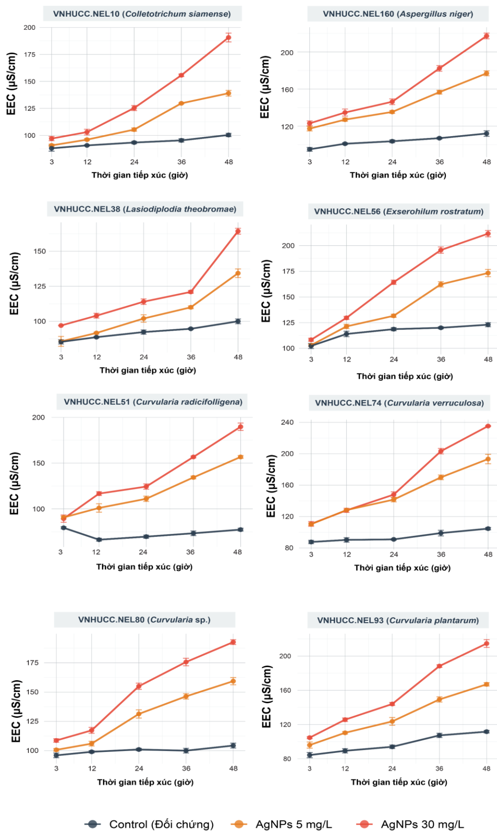
Hình 3.31. Sự biến động giá trị EEC quan sát được theo thời gian của từng phân lập thử nghiệm. Độ lệch chuẩn (SD) được biểu thị tại các nút mang dữ liệu tương ứng.
