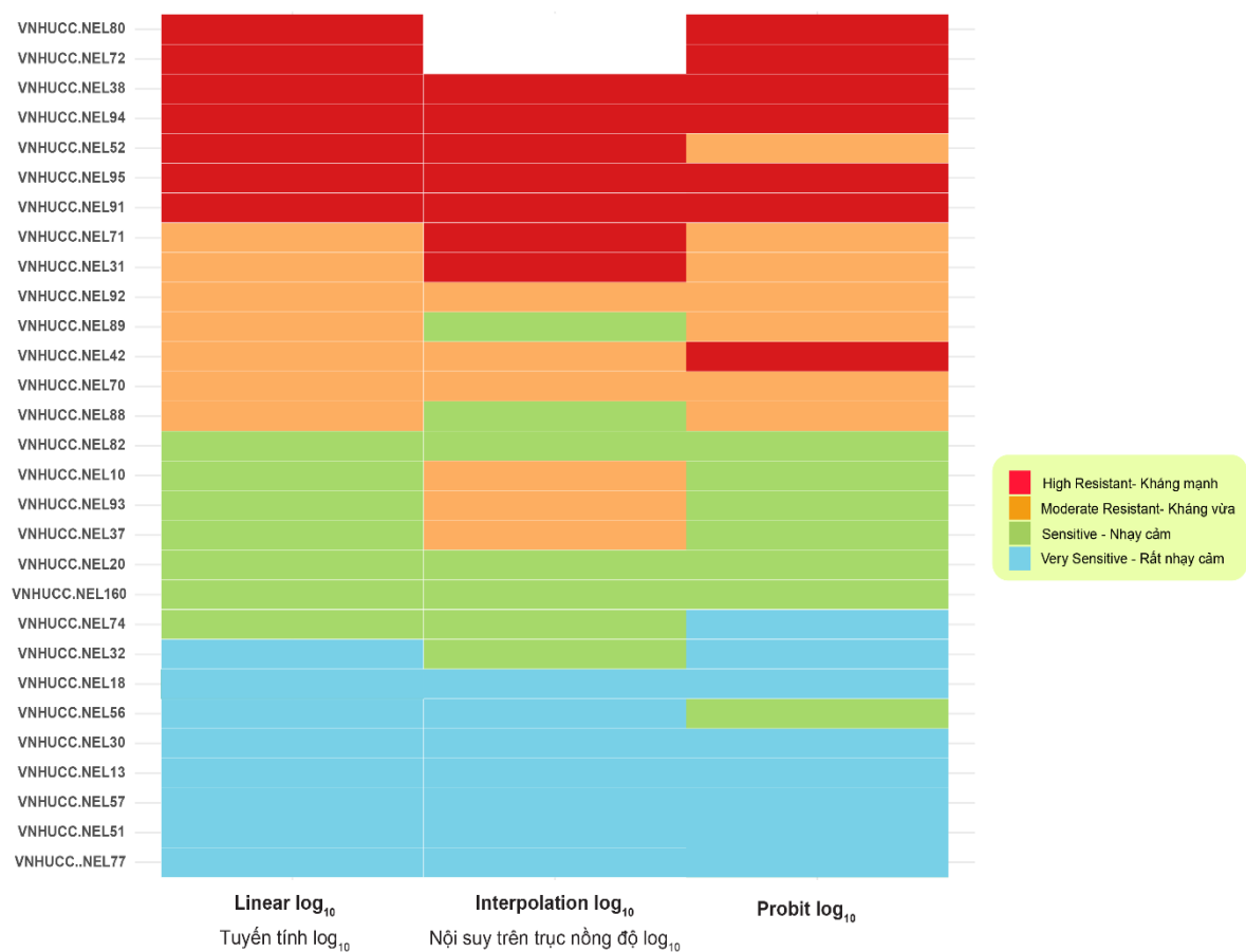
Phụ lục Hình 4.9. Sự khác biệt trong phân bố mức độ nhạy cảm của các chủng phân lập theo dữ liệu giá trị ước tính EC_{50} tương ứng với các mô hình ước tính khác nhau
