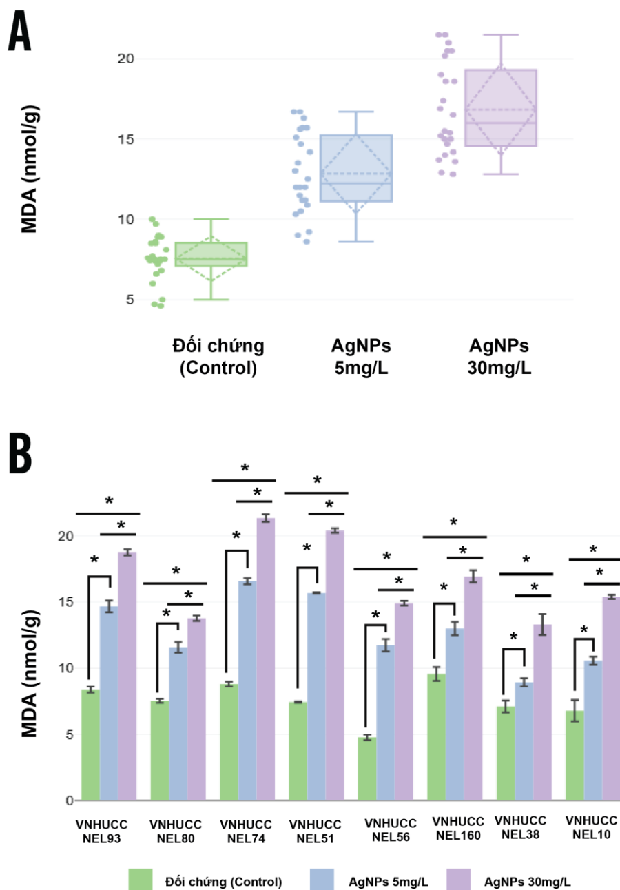
Hình 3.33. Hàm lượng MDA ( \mu\text{mol/g} ) khi xử lý với nano bạc sau 48 giờ. A. Biểu đồ phân bố (Box plot) các giá trị dữ liệu quan sát được của MDA giữa nhóm đối chứng (Control) và nhóm được xử lý với nano bạc (5 mg/L và 30 mg/L). B. Biểu đồ cho thấy sự khác nhau hàm lượng MDA theo từng phân lập. Độ lệch chuẩn (SD) được biểu thị tại các cột mang dữ liệu tương ứng. Sự khác biệt có ý nghĩa ( p < 0,05 ) được biểu thị bằng “*”. từng phân lập.
