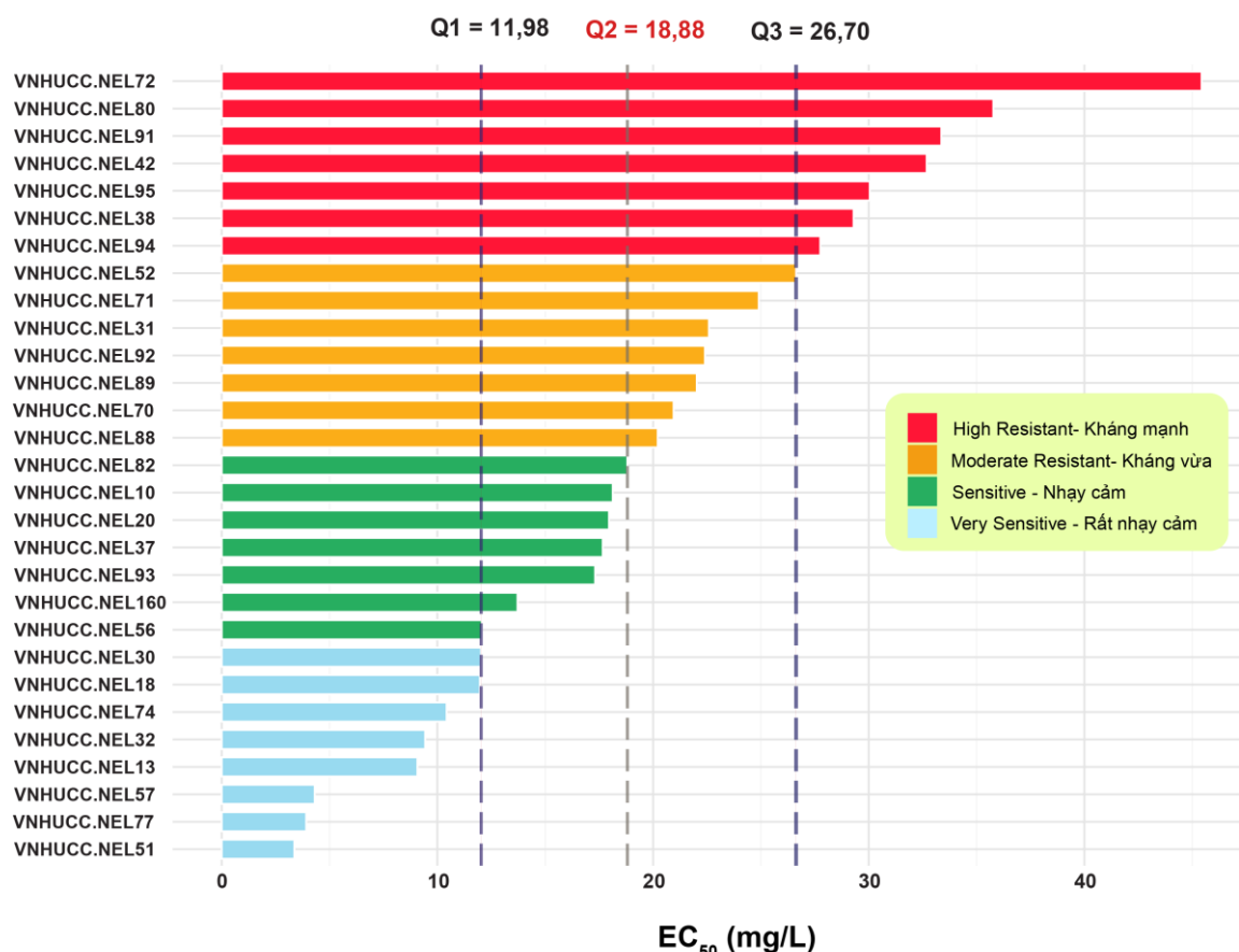
Hình 3.17. Sự phân bố các giá trị EC_{50} của các chủng phân lập thử nghiệm theo mô hình Probit \log_{10} . Mức độ nhạy cảm của các chủng phân lập với nano bạc được phân nhóm bằng phương pháp thống kê mô tả tứ phân vị dựa trên 3 điểm ngưỡng (Q1, Q3 – đường đứt nét màu xanh, Q2 – giá trị trung vị - đường đứt nét màu xám). Các nhóm mức độ nhạy cảm khác nhau với nano bạc được thể hiện bằng các khối màu tương ứng.
