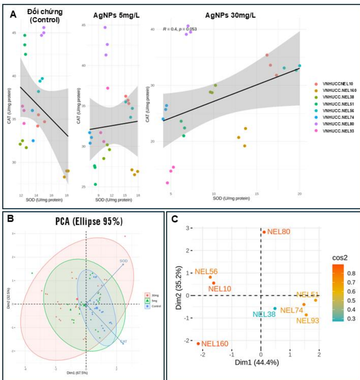
Phụ lục Hình 4.10. Mối tương quan giữa hai enzyme SOD và CAT và sự phân bố đáp ứng của chủng phân lập khi xử lý với nano bạc ở các nồng độ khác nhau. (A). Mức độ tương quan của 2 enzyme (B). Biểu đồ PCA (Ellipse với độ tin cậy 95%) theo tác động của các công thức xử lý (Màu hồng cam – AgNPs 30 mg/L, màu lục – AgNPs 5 mg/L và màu xanh dương – Đối chứng) (C). Biểu đồ PCA theo chủng phân lập. Màu sắc phản ánh giá trị \cos^2 (mức độ đóng góp của từng mẫu vào các chiều PCA). Màu cam (giá trị \cos^2 cao) thể hiện các mẫu có đóng góp lớn vào các thành phần chính, trong khi màu xanh (giá trị \cos^2 thấp) thể hiện đóng góp thấp hơn.
